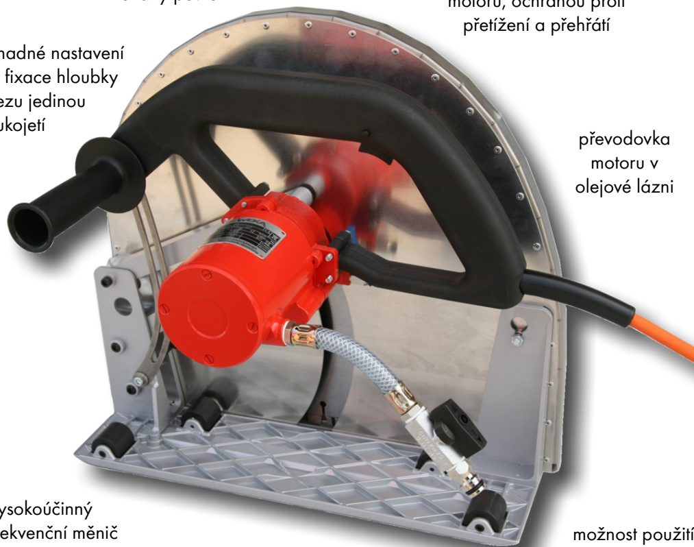
mechanika ponoření kotouče
